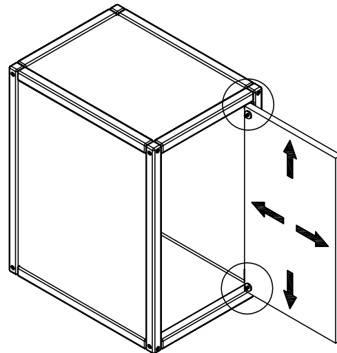
C ...stellen Sie sich die Tür wie gewünscht ein.
